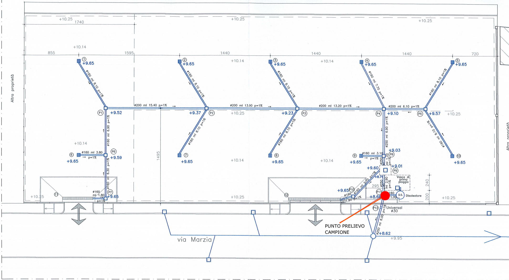
PLANIMETRIA IMPIANTO DI FOGNATURA Scala 1:200
